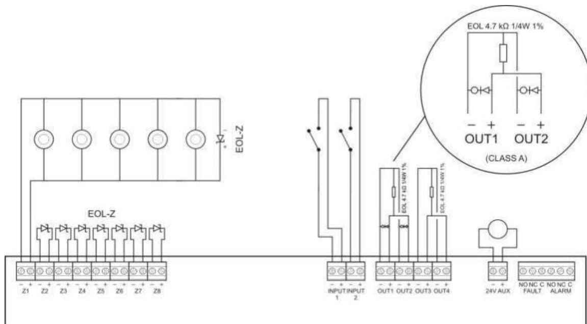
Bild 5: EN 54-13 brandsystemanslutningar
