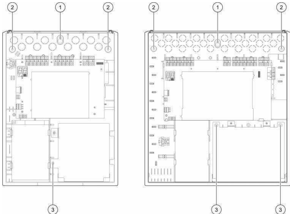
Bild 3: Skruvhålens placering
